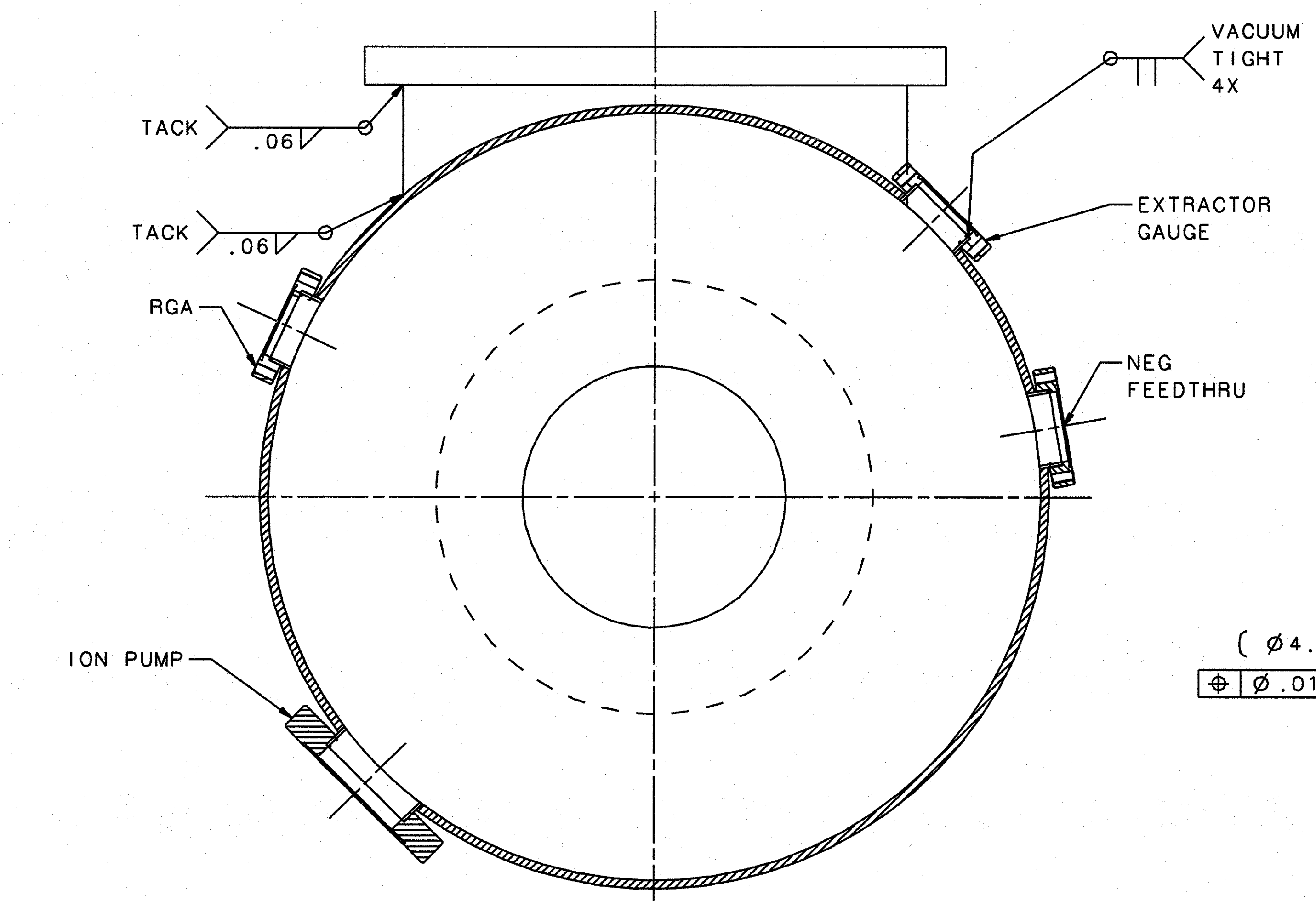
SECTION A-A
