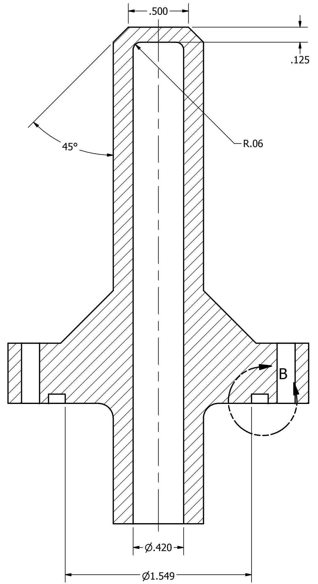
SECTION A-A SCALE 2 : 1
