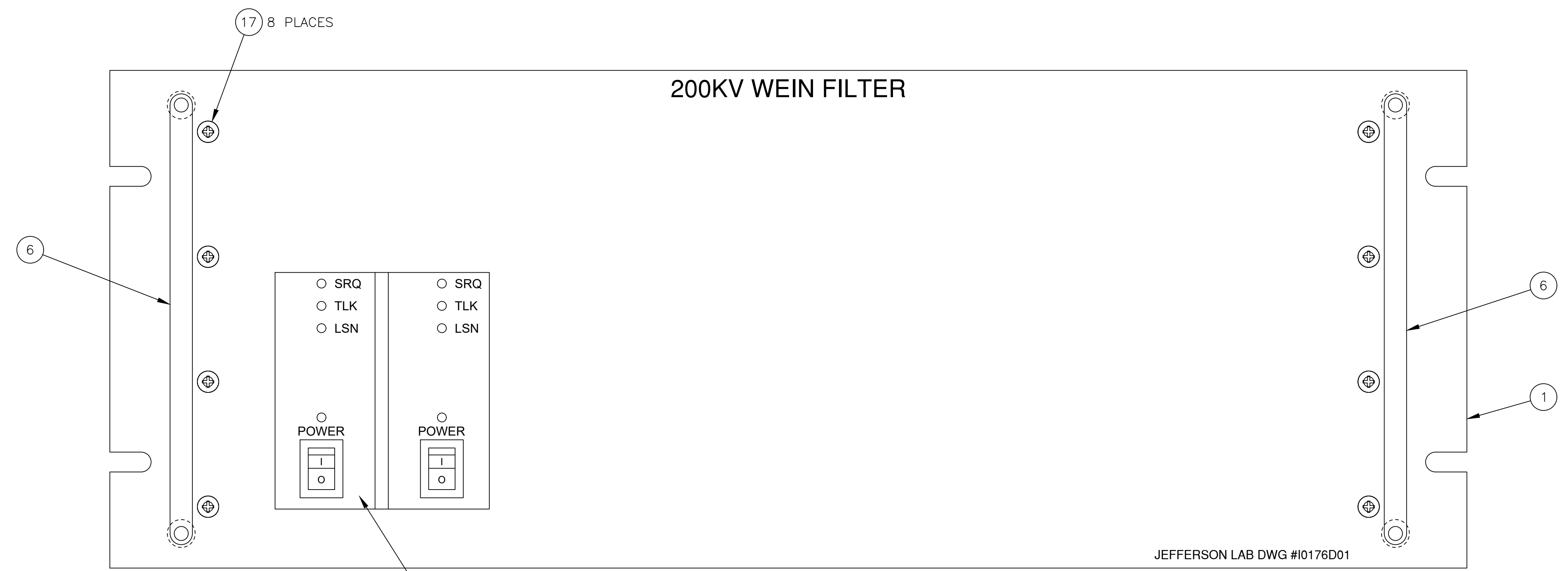
VIEW A-A
