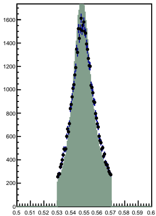
Mass( eta )
