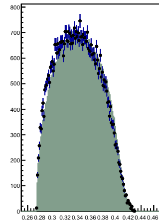
Mass( PI- PI0 )
