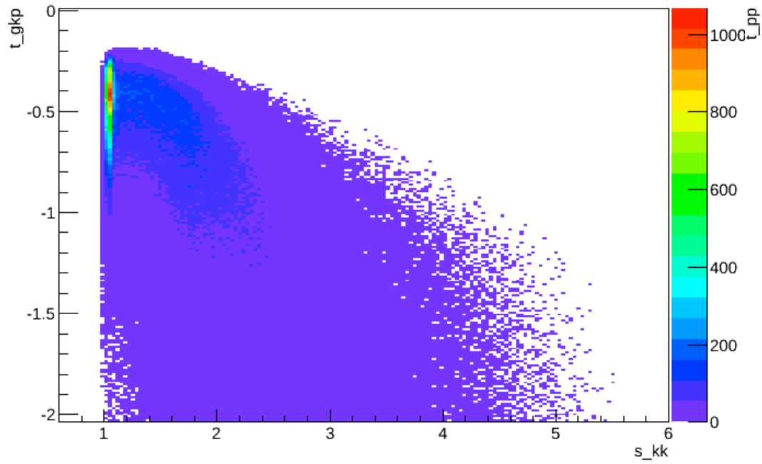
t_gkp:s_kk {s_gp>9.4}
