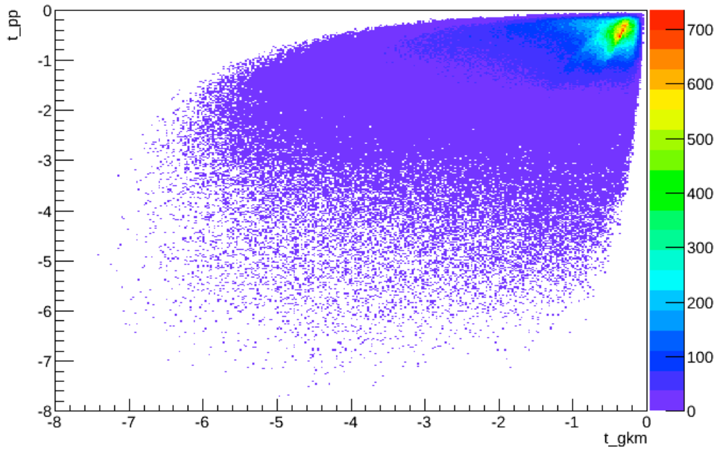
t_pp:t_gkm {s_gp>9.4}
