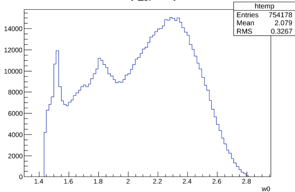
w0 {s_gp&gt;9.4}
