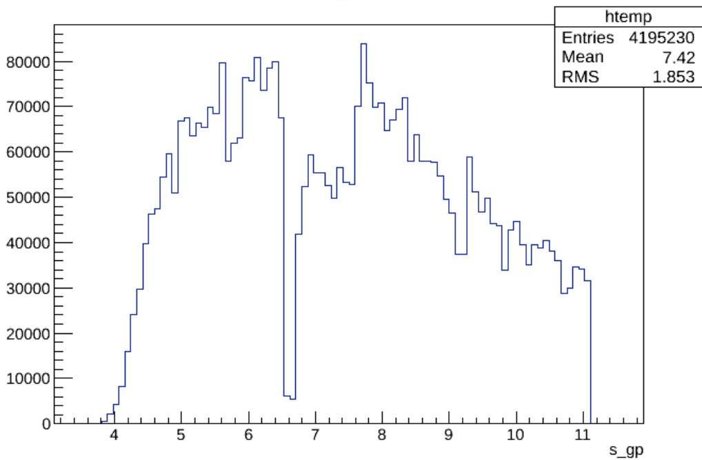
s_gp
