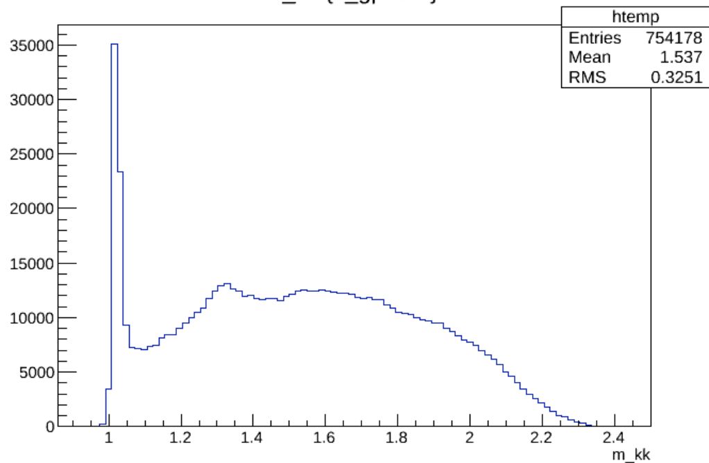
m_kk {s_gp&gt;9.4}
