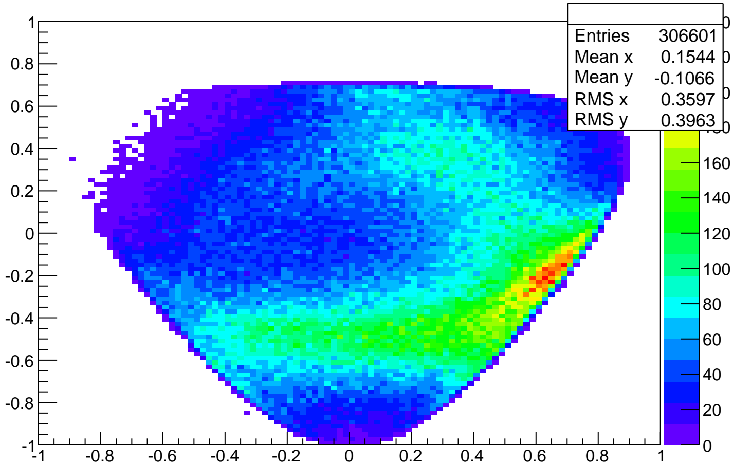
Dalitz_y_cb: Dalitz_x_cb {mm_PPipPim_cb < 0.14}
