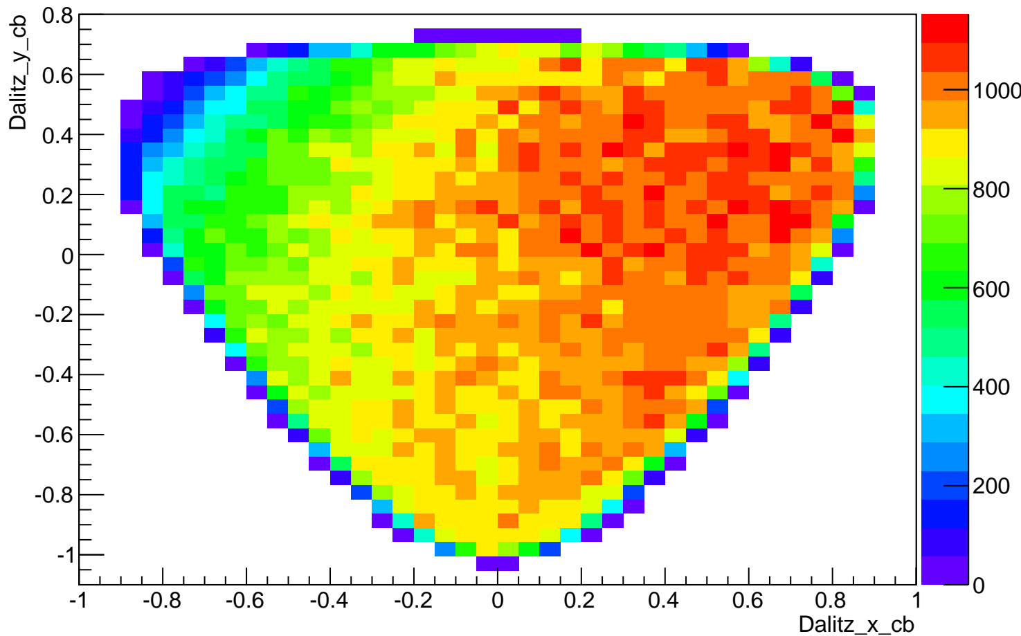
Dalitz_y_cb:Dalitz_x_cb
