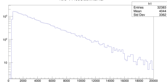
10.0*V1495ClockInterval
